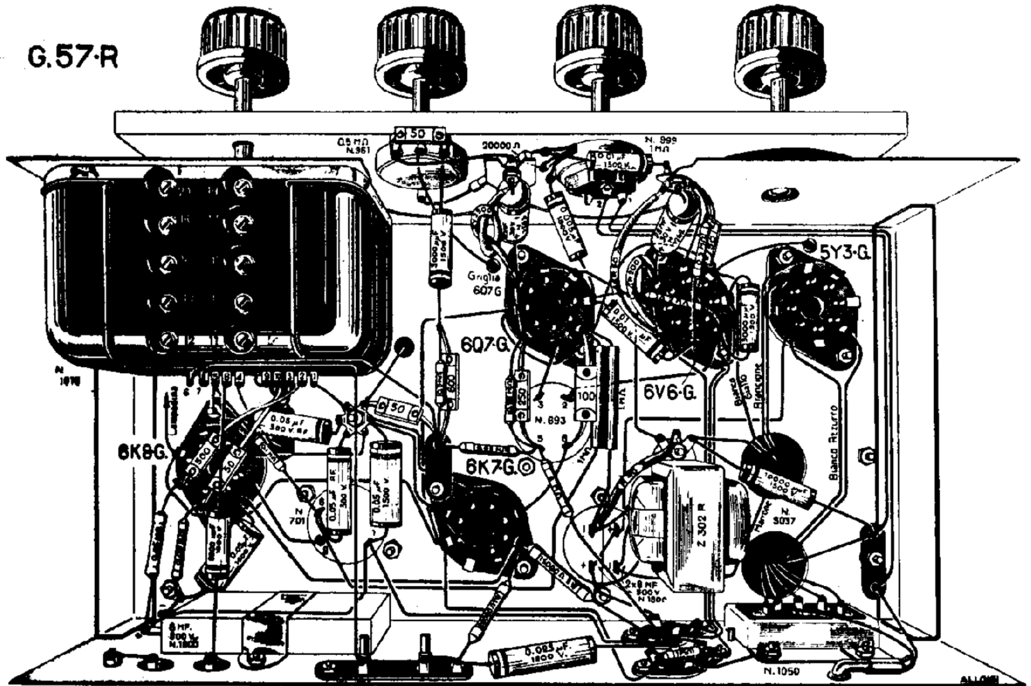
Il piano costruttivo del « G 57 R ».
